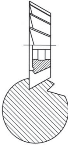
Tek Açılı Konik Freze
